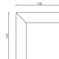
Kotni element T-C-115/115
