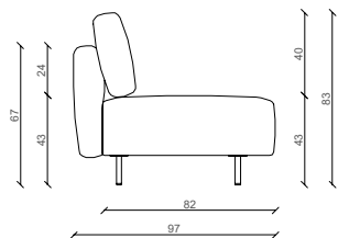
Stranski prikaz
