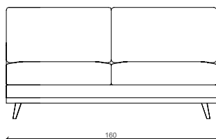
Zaključni element H-E-160
